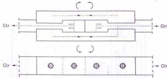
Gambar 12.20 Sambungan Memanjang Balok Kunci Jepit
