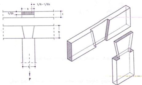
Gambar 12.25 Hubungan Ekor Burung Layang
