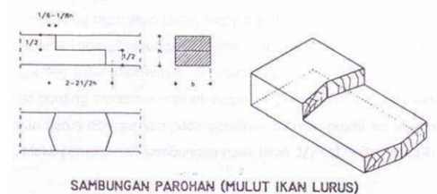
Gambar 12.15 Sambungan Bibir Lurus
