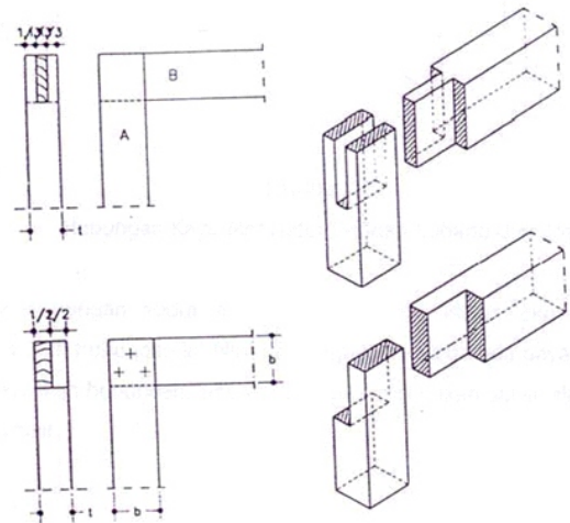
12.22 Hubungan Kayu Menyudut.
