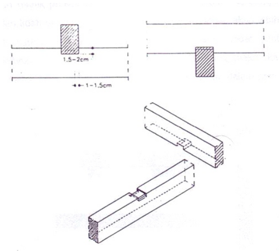
Gambar 12.31 Hubungan Loef dan Voorloef
