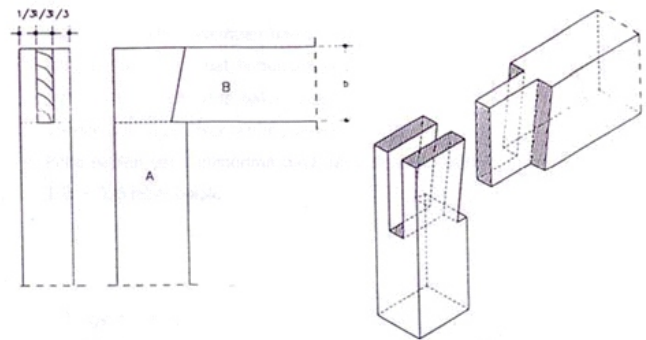
Gambar 12.23 Hubungan Kayu Menyudut Dengan Lubang dan Gigi
