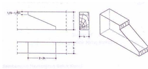
Gambar 12.17 Sambungan Bibir Miring
