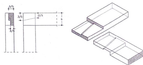
Gambar 12.24 Hubungan Ekor Burung terbenam
