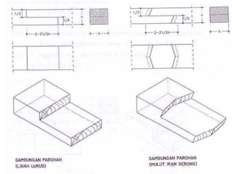
Gambar 12.14 Sambungan Bibir Lurus
