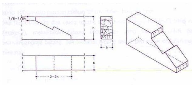
Gambar 12.18 Sambungan Bibir Miring Berkait
