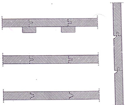
Gambar 12.32 Sambungan Kayu Arah Melebar
