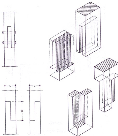
Gambar 12.21 Sambungan Memanjang Tegak Lurus Hubungan Kayu
