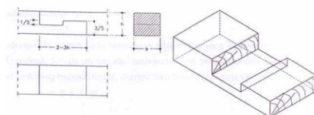
Gambar 12.16 Sambungan Bibir Lurus Berkait
